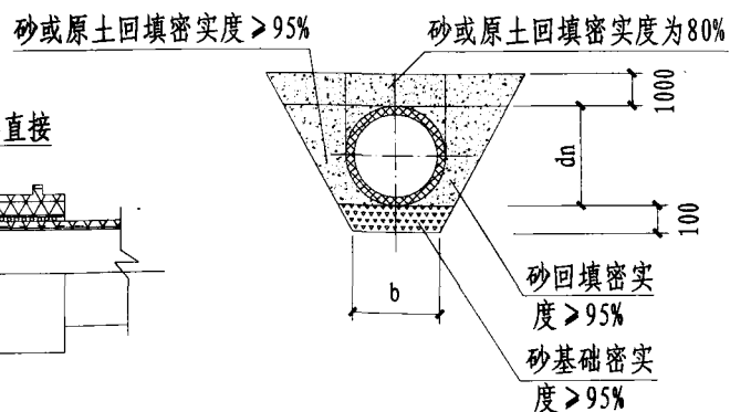
直埋或直埋穿越车行道
