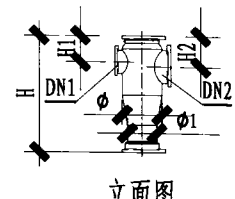
立面图
