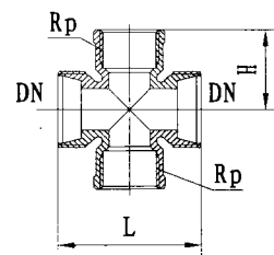
内螺纹四通
