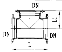
等径三通
