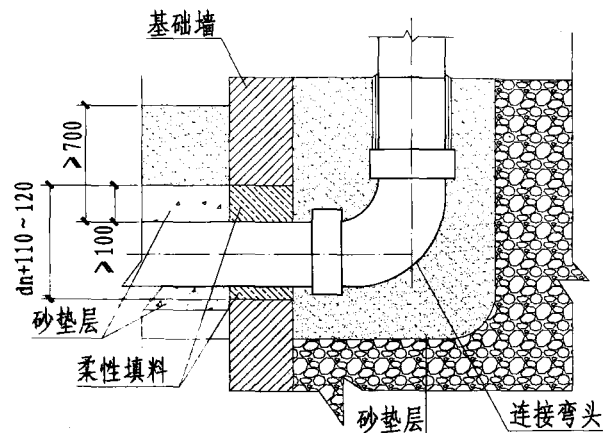
穿基础墙
