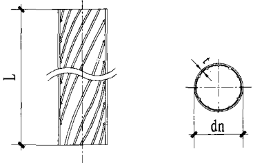
PVC-U加强型内螺旋管
