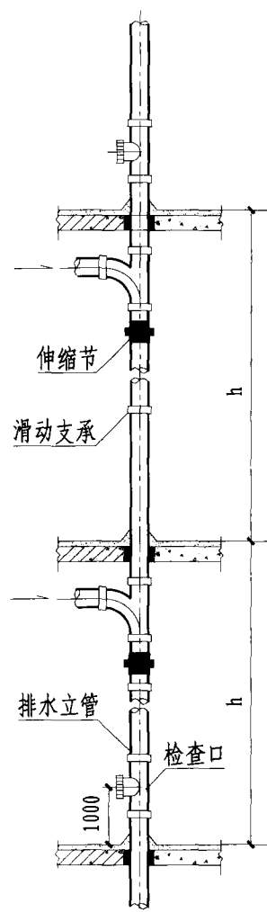
单立管
