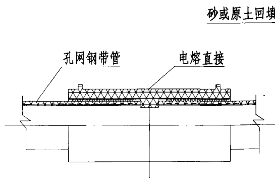
电熔直接连接
