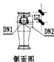
侧面图
