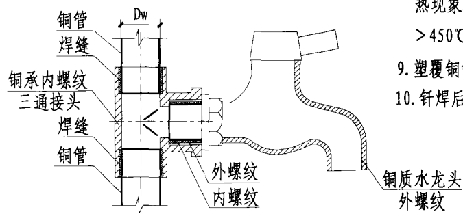
管材与管配件连接
