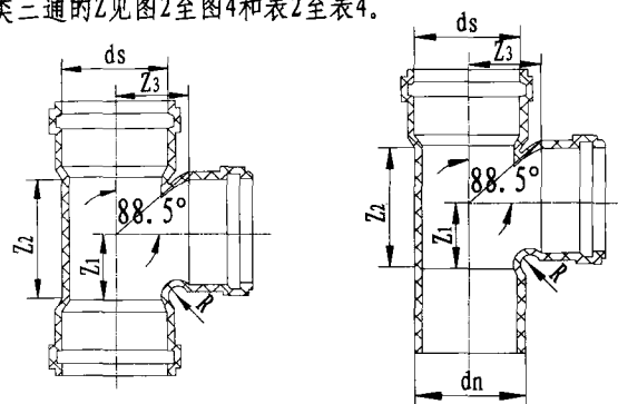
a) 顺水三通
