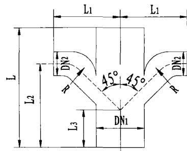
W型
