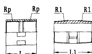
内螺纹直通 外螺纹直通 双内螺纹直通
