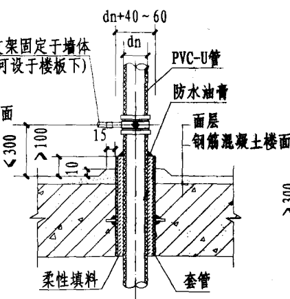
穿楼面 (四)
