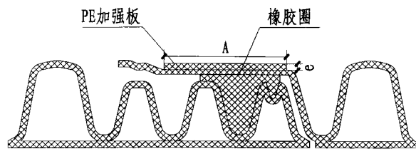
连接示意图
