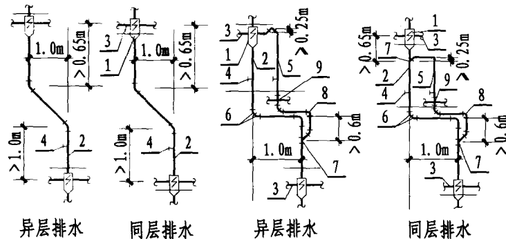
图3 偏置距离 \leq 1\text{m} 时, 45°弯头连接方式
