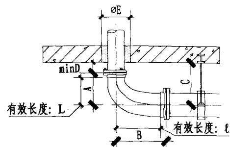
STD型底部弯头
