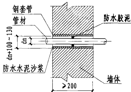
穿内墙
