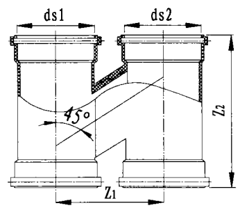
图8 H型管件
