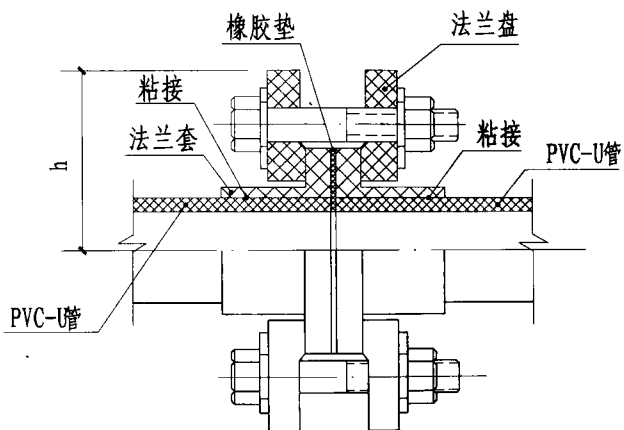
法兰连接
