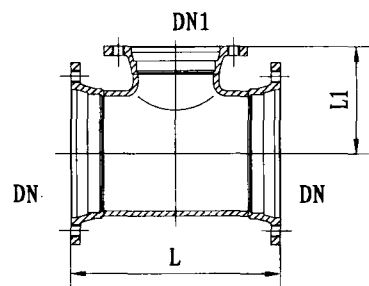
法兰-法兰
