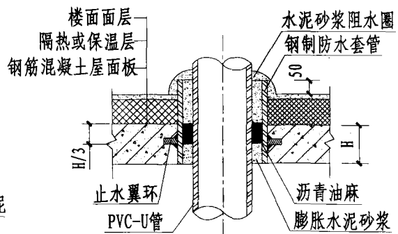
穿屋面板
