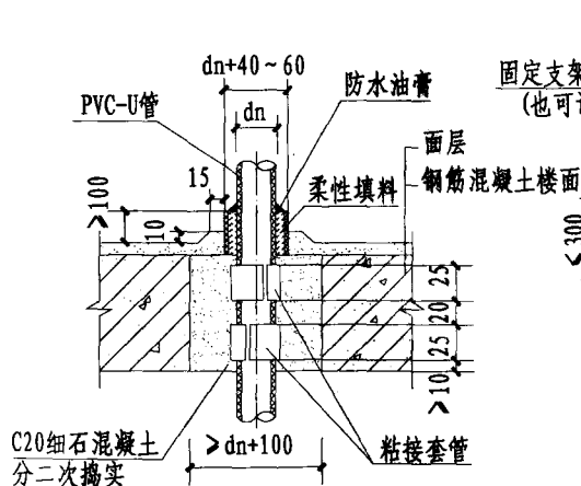
穿楼面 (三)
