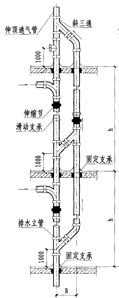
I 型
