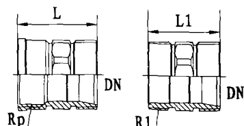
内螺纹直通 外螺纹直通 双内螺纹直通
