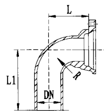
A型
