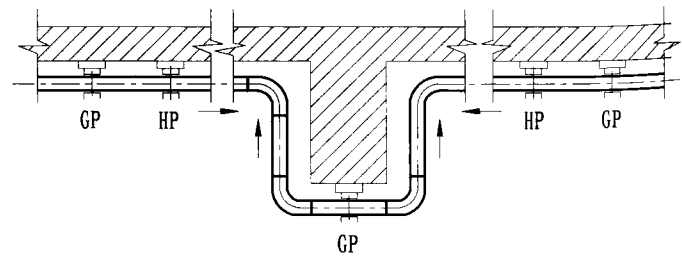
U形补偿
