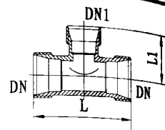
异径支流三通
