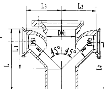
A型
