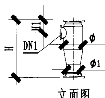
立面图
