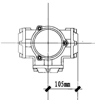
五通加强型接头 型号: C-5005
