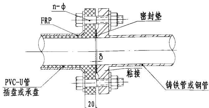
法兰连接
